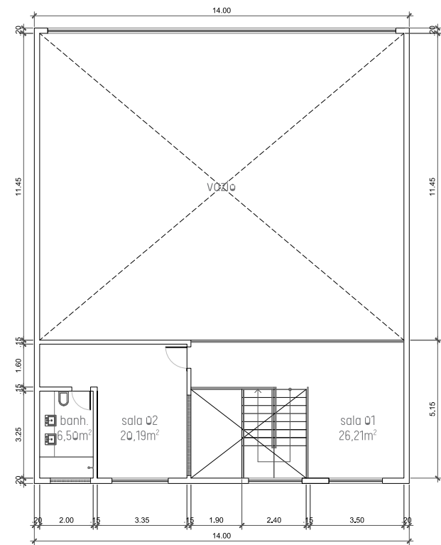
planta baixa mezanino
