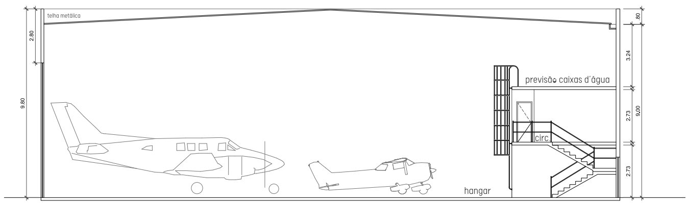
corte BB
