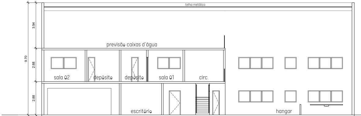
corte AA
