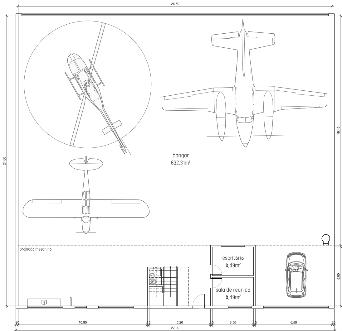
planta baixa pav. térreo
