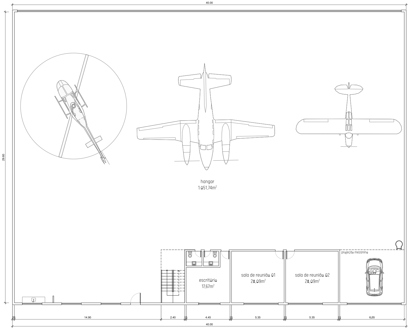
planta baixa pav.térreo
