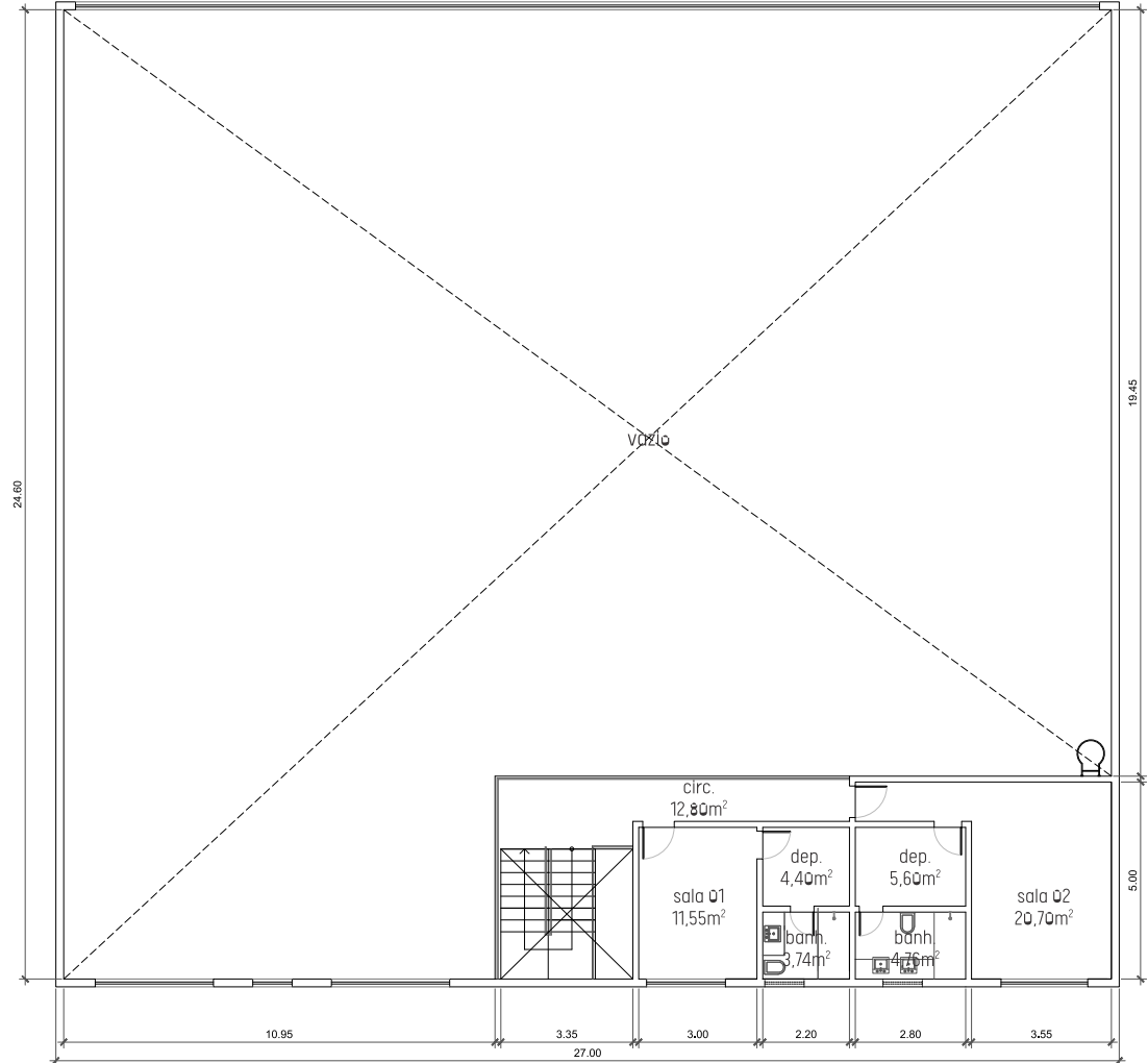
planta baixa mezanino
