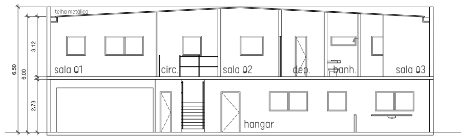
corte AA
