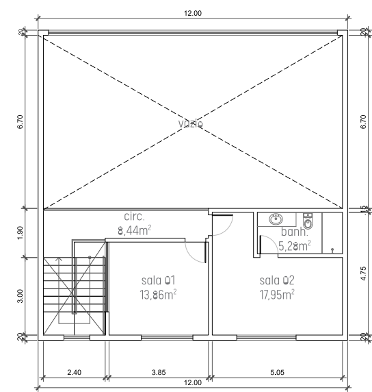
planta baixa mezanino
