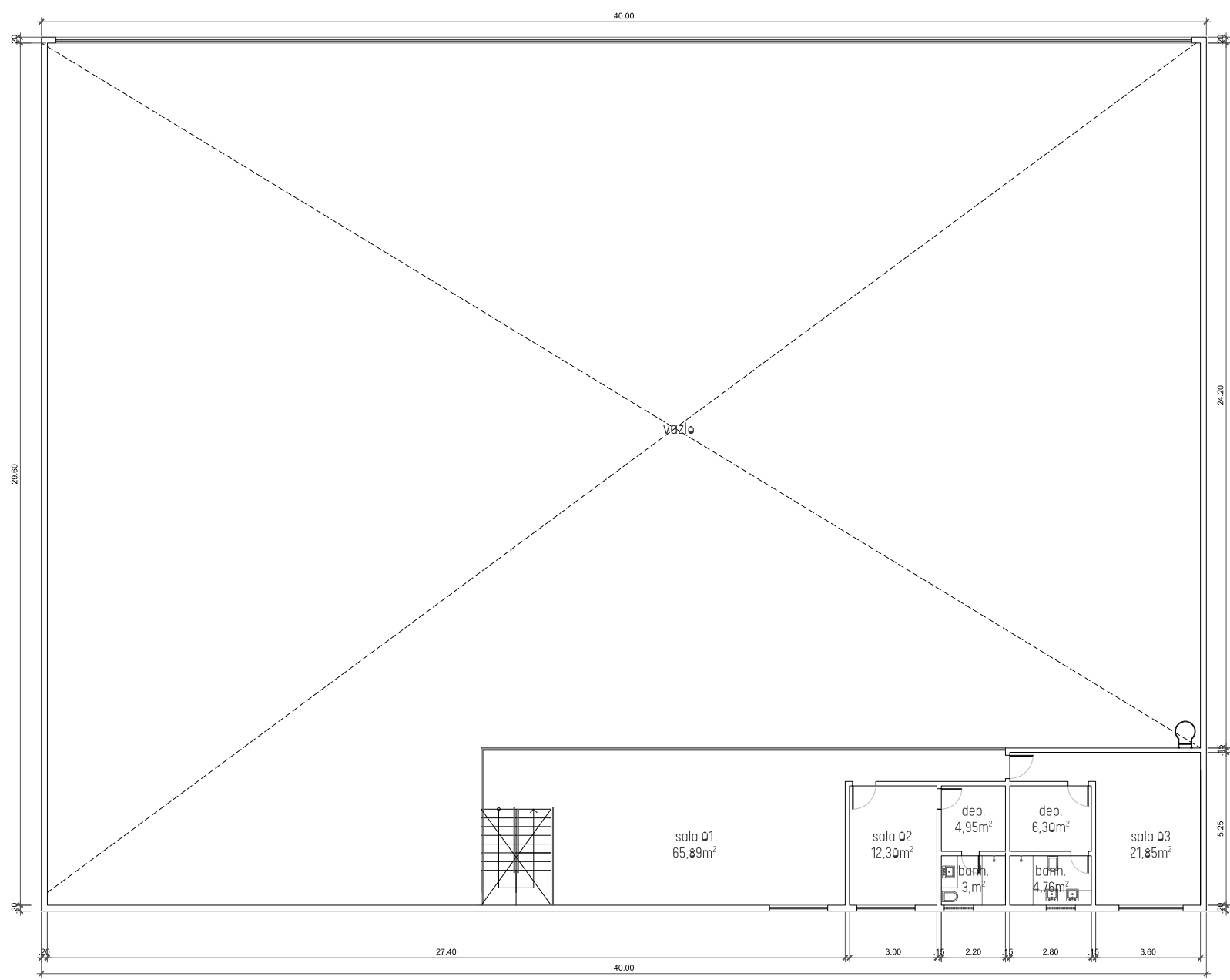
planta baixa mezanino
