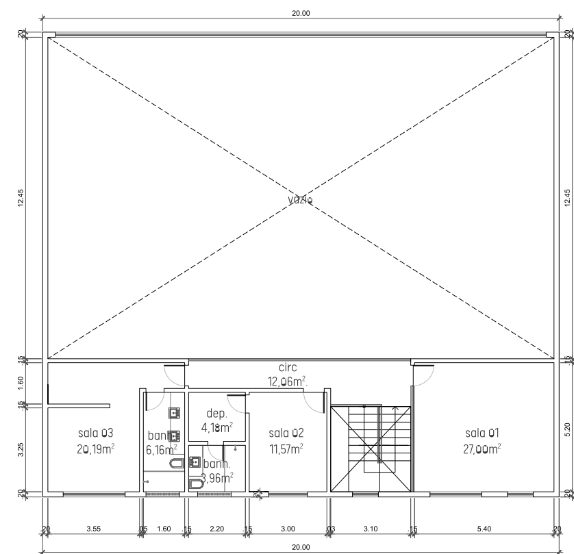
planta baixa mezanino
