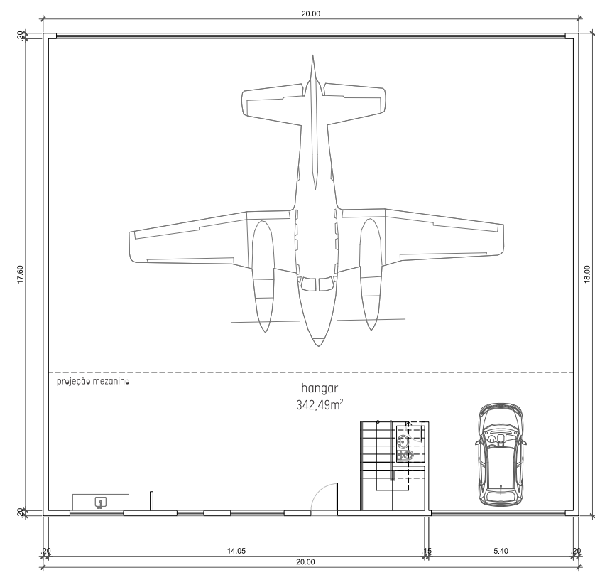
planta baixa pav.térreo
