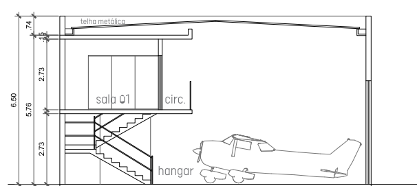
corte BB
