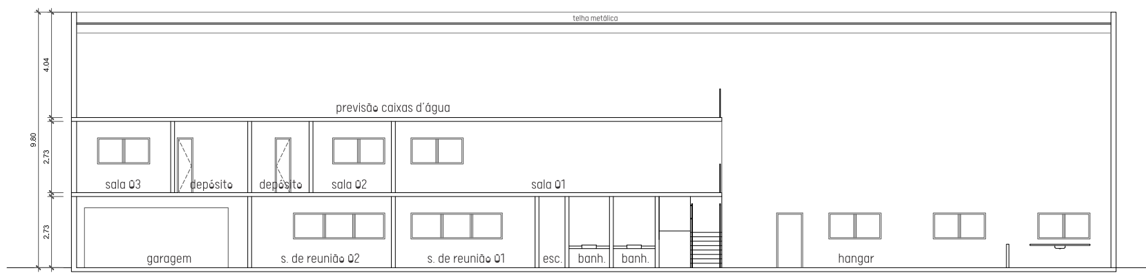
corte AA
