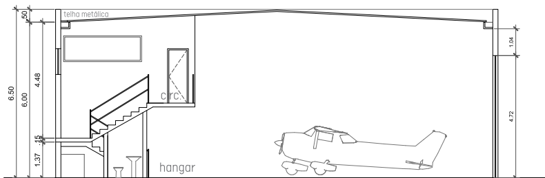
corte BB
