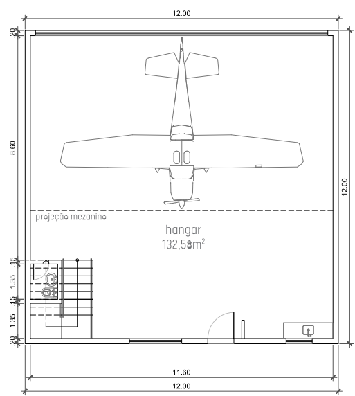
planta baixa pav. térreo
