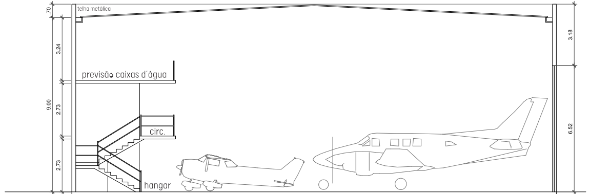
corte BB
